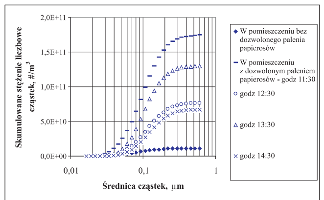
Rys. 4. Skumulowane stężenie liczbowe cząstek (SMPS) występujących w powietrzu w pomieszczeniu bez/z dozwolonym paleniem papierosów
