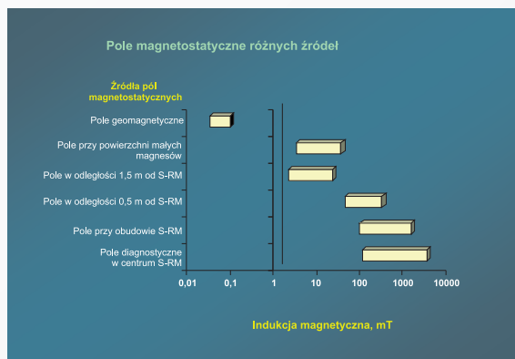
Rys. Z1. Pola magnetostaticzne wytwarzane przez różne źródła
