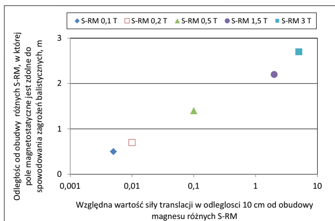
Rys. Z3. Względna wartość siły transjacji wywieranej na obiekty ferromagnetyczne i zasięg pola magnetycznego wywołującego zagrożenia balistyczne w otoczeniu magnesów różnego typu S-RM
