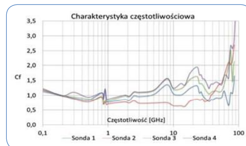
Rys. 6. Charakterystyki częstotliwościowe komercyjnych sond pomiarowych w paśmie 0,1-90 GHz. ( C_f – częstotliwościowy współczynnik korekcyjny)
