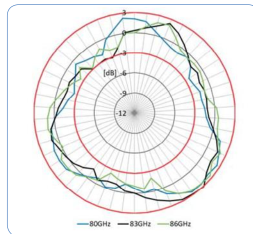
Rys. 7. Izotropowość sondy 1 pola elektrycznego w Paśmie E
